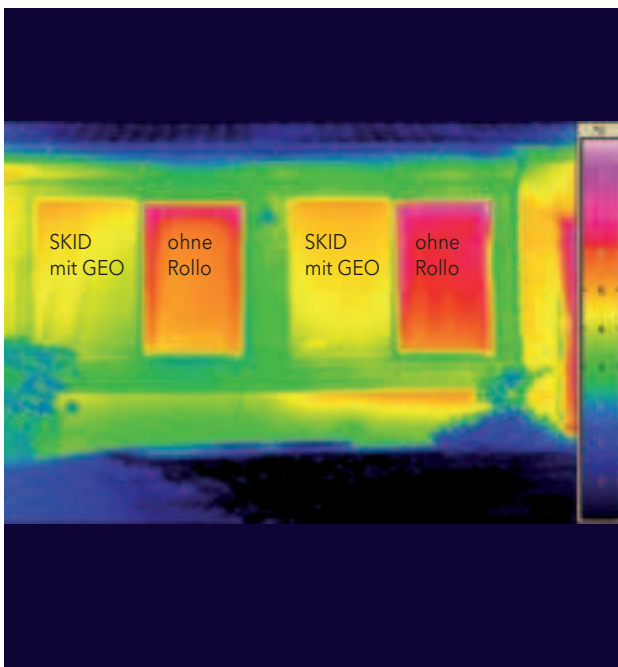
Thermografie-Aufnahme im Winter. Der Wärmeverlust am Fenster ohne Rollo ist gut zu erkennen.
