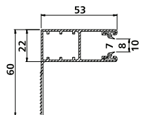
CR 53 Sonderführungsschiene mit Winkel, z.B. für Rechtsrollermontage (wird ohne Bohrung ausgeliefert)
