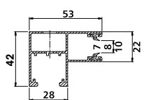
CA 53* Distanzführungsschiene für Kastengröße 165, 180 und 205 mm (150er Kasten auf Anfrage)
