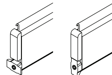
Endleistenanschlag, drehbar* für einfachen Panzertausch
