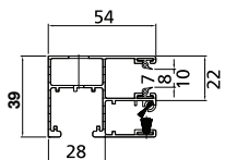
CI 53* Insektenschutzführungsschiene (vgl. Baubarkeiten Insektenschutz-Rollo)
