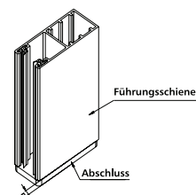
CA 53* Distanzführungsschiene für Kastengröße 165, 180 und 205 mm (150er Kasten auf Anfrage)
